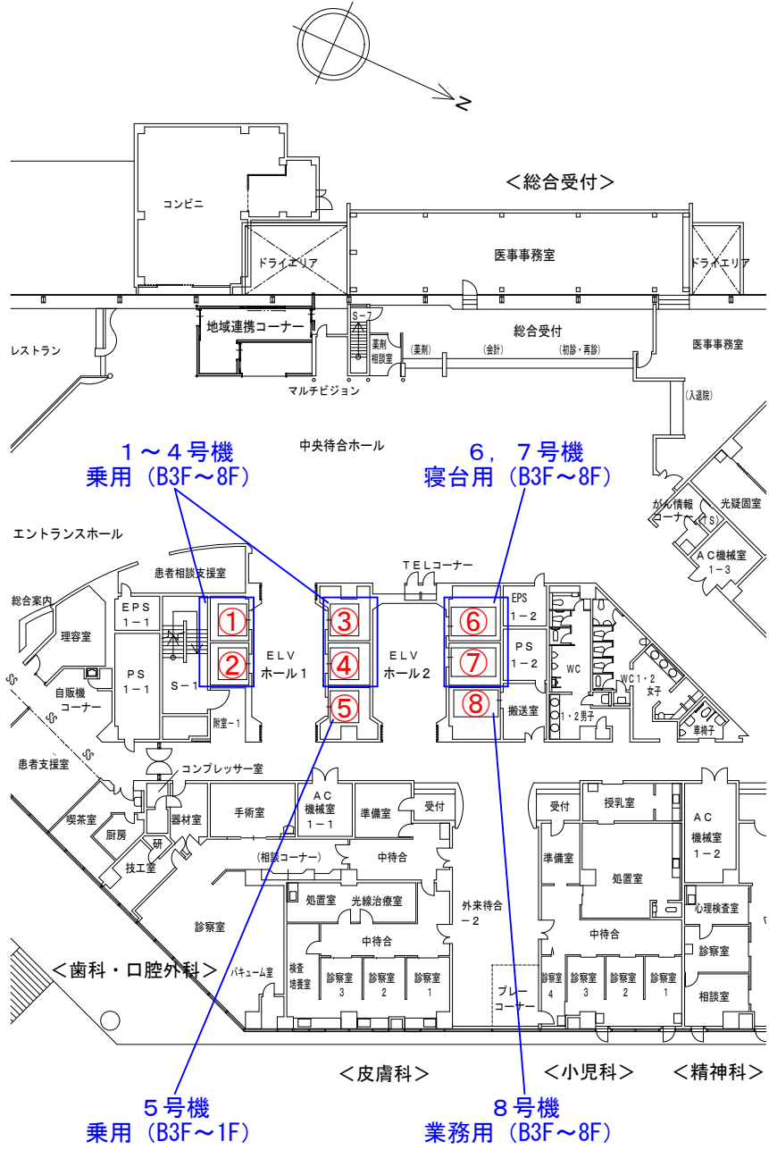
病棟側 (1 ~ 8 号機)
