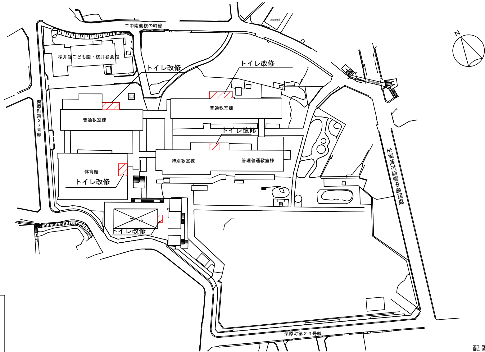
配置図
