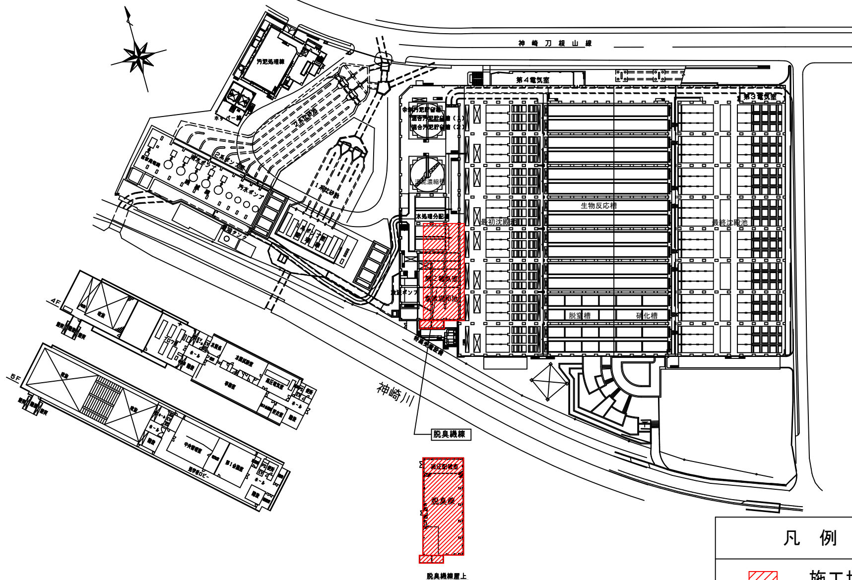
豊中市庄内下水処理場一般平面図
