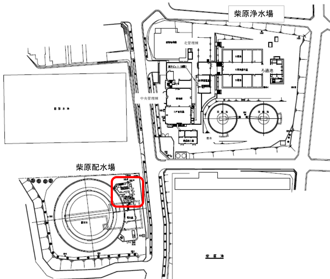
柴原浄配水場 一般平面図
