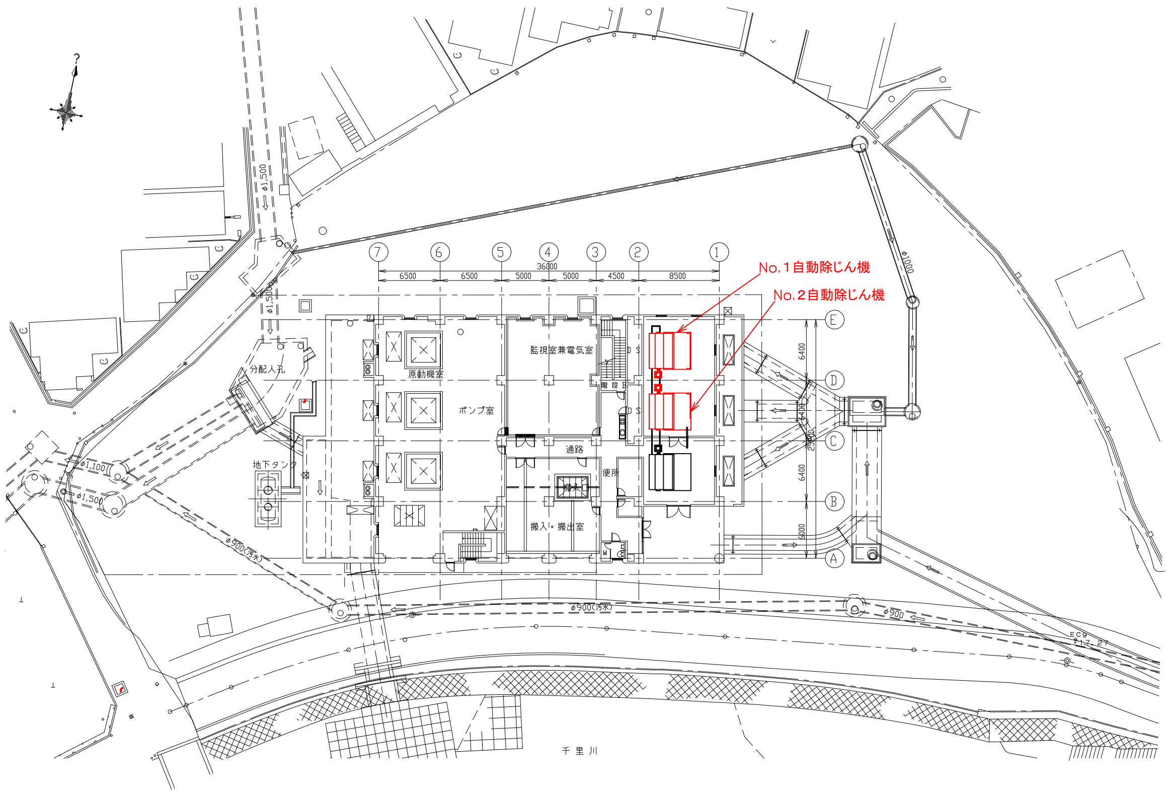
千里園ポンプ場 一般平面図
