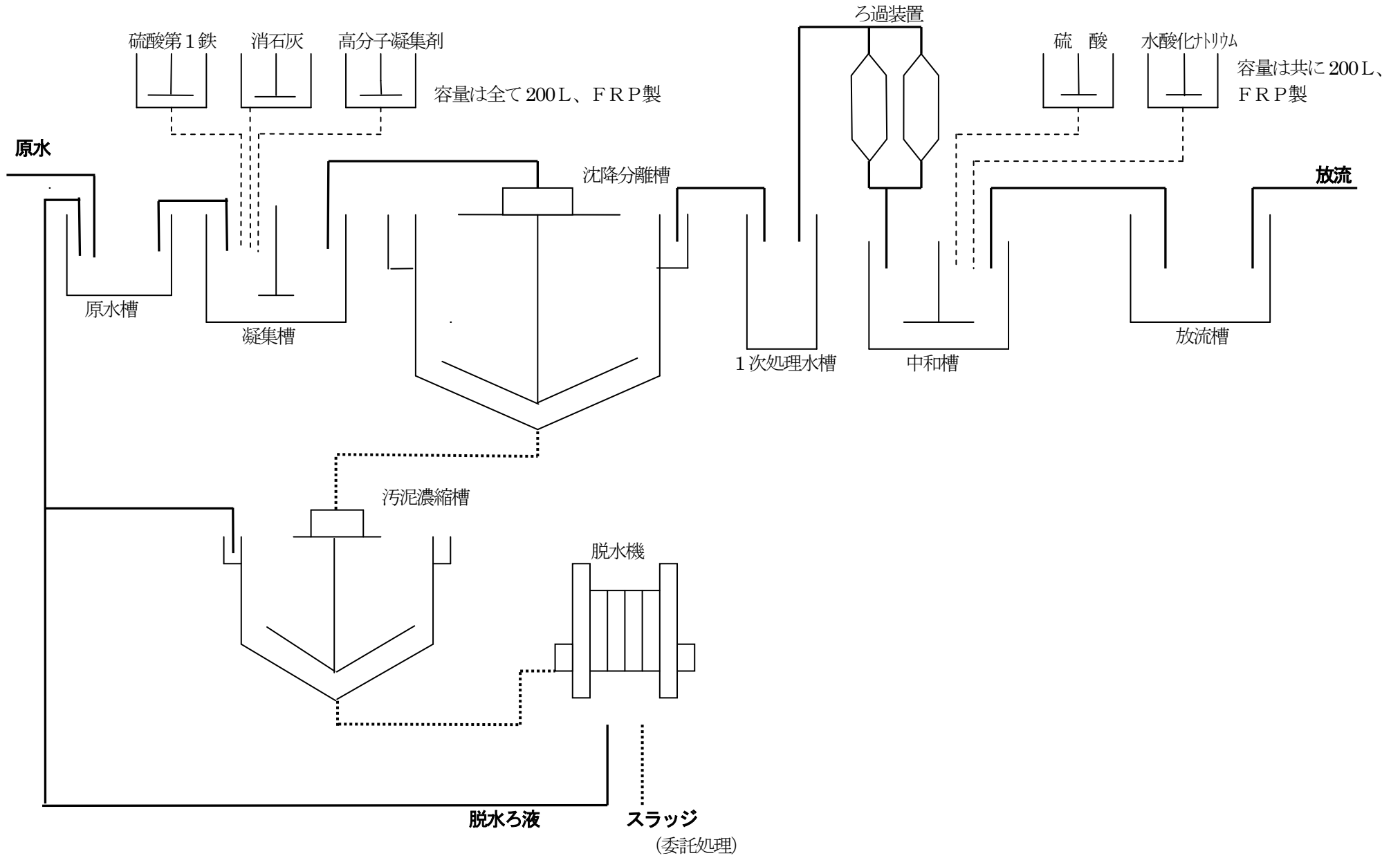
別図4 汚水処理施設の処理系統図 注) 処理施設の仕様書、設計図面等を添付すること。
