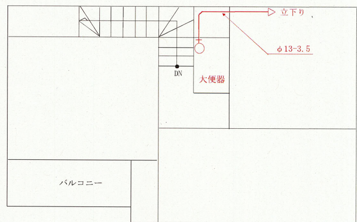
(2 階平面図)
