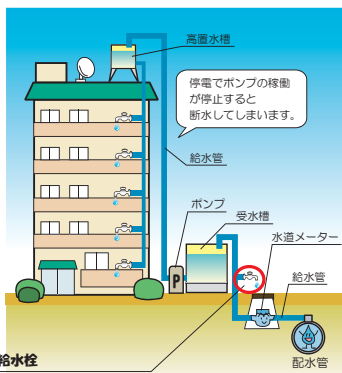
受水槽式給水
