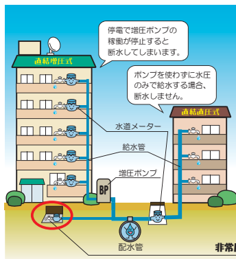
直結式給水
