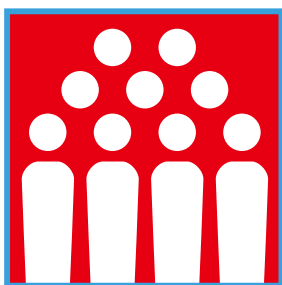
密集回避
