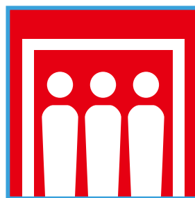
密室回避
