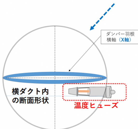
温度ヒューズの設置位置（ダクト内下部）
