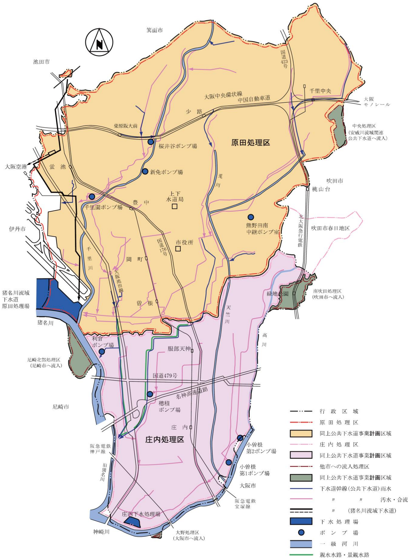
図1-11 排水系統図
