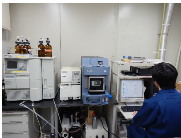
写真 2 高速液体クロマトグラフ質量分析計
