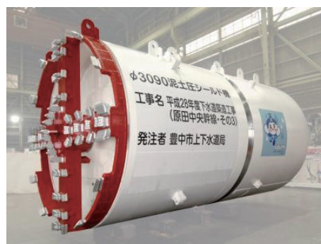
▲ 下水道を設置するための掘削機（シールドマシン）
