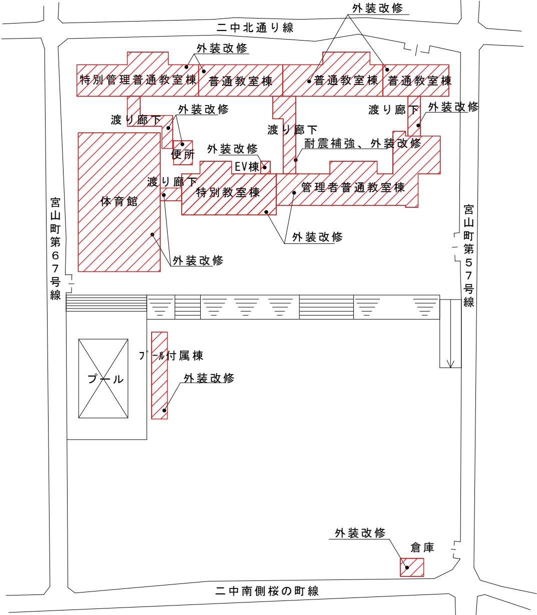
配置図
