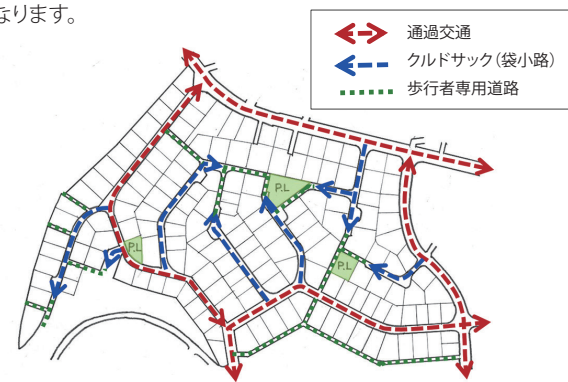
戸建て住宅地に導入されたラドバーン方式の例
